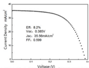
(b) 3 階段硒化法之 CZTSe 太陽能電池的 I-V 曲線
